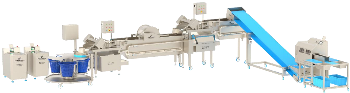
HS-FLEX dans une ligne de transformation de légumes pour couper, laver et sécher des légumes
