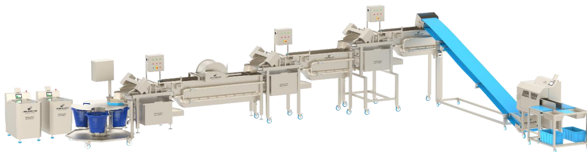
HCB-400-TS extendida para lavado en 3 etapas
