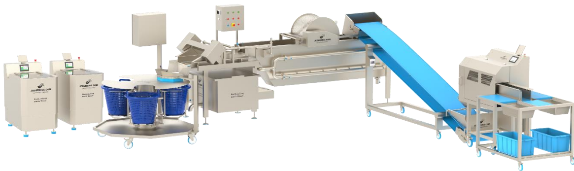
HCB-400-TS en una línea de procesamiento de verduras para lavar, cortar y secar verduras
