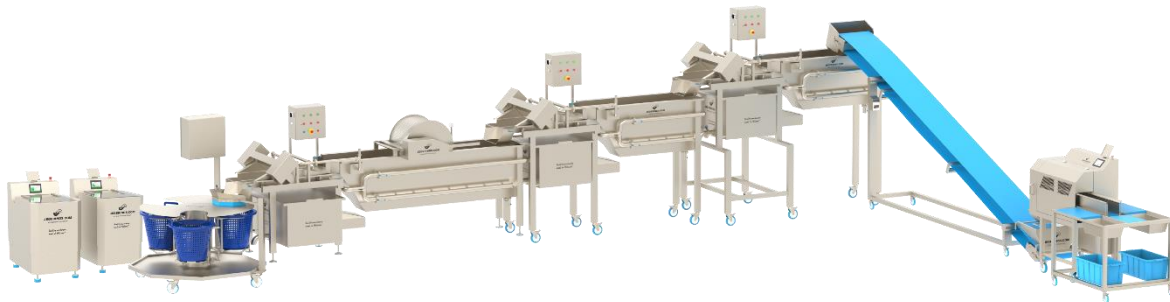
HCB-400-TS verlengd voor een 3-fase wassysteem
