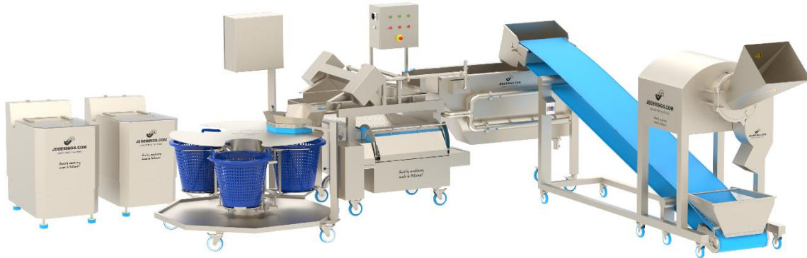
Die 3DD Würfelschneidemaschine in einer Gemüseverarbeitungslinie zum Schneiden, Waschen, (Sortieren) und Trocknen von Gemüse
